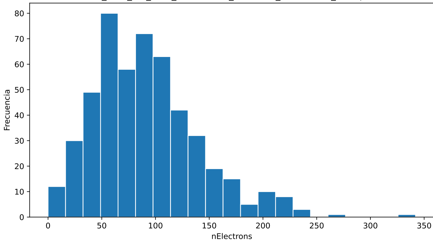
Distribución de nElectrons ar_90.0_cf4_10.0_110.0kVcm_1.000bar_0.0204mm_500npe
