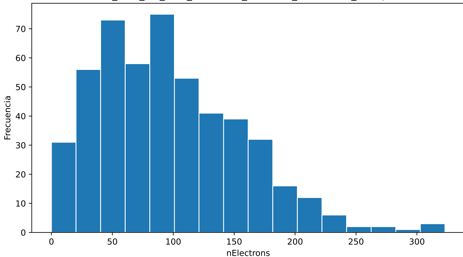
Distribución de nElectrons ar_90.0_cf4_10.0_60.0kVcm_1.000bar_0.0473mm_500npe
