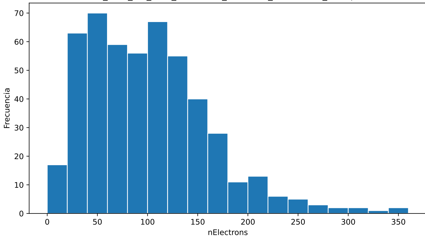
Distribución de nElectrons ar_90.0_cf4_10.0_70.0kVcm_1.000bar_0.0378mm_500npe
