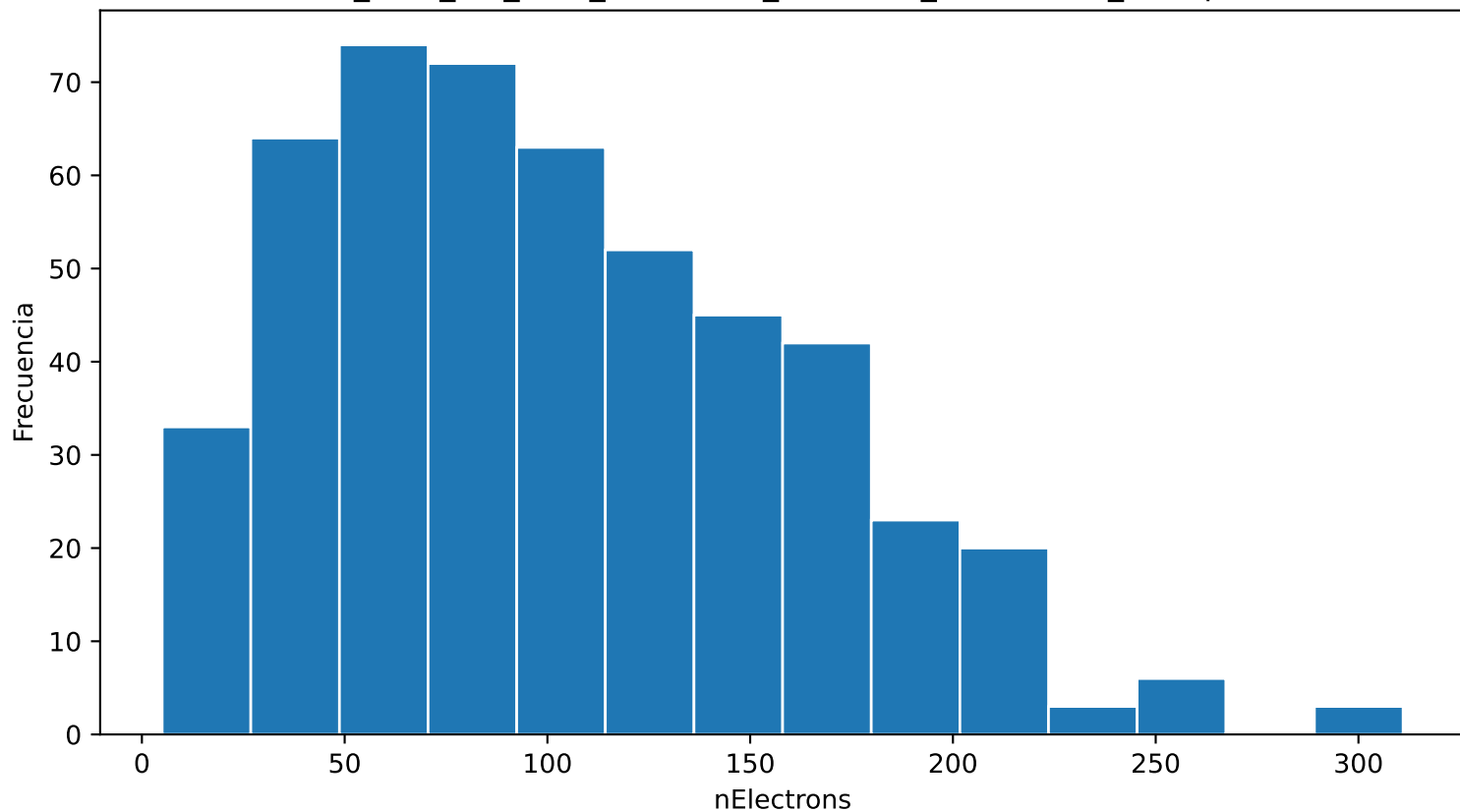
Distribución de nElectrons ar_90.0_cf4_10.0_80.0kVcm_1.000bar_0.0313mm_500npe
