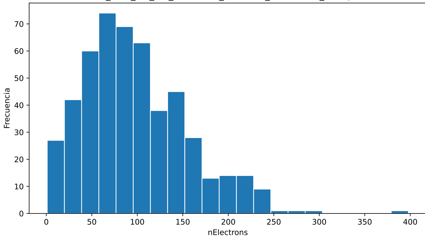
Distribución de nElectrons ar_95.0_cf4_5.0_70.0kVcm_1.000bar_0.0369mm_500npe
