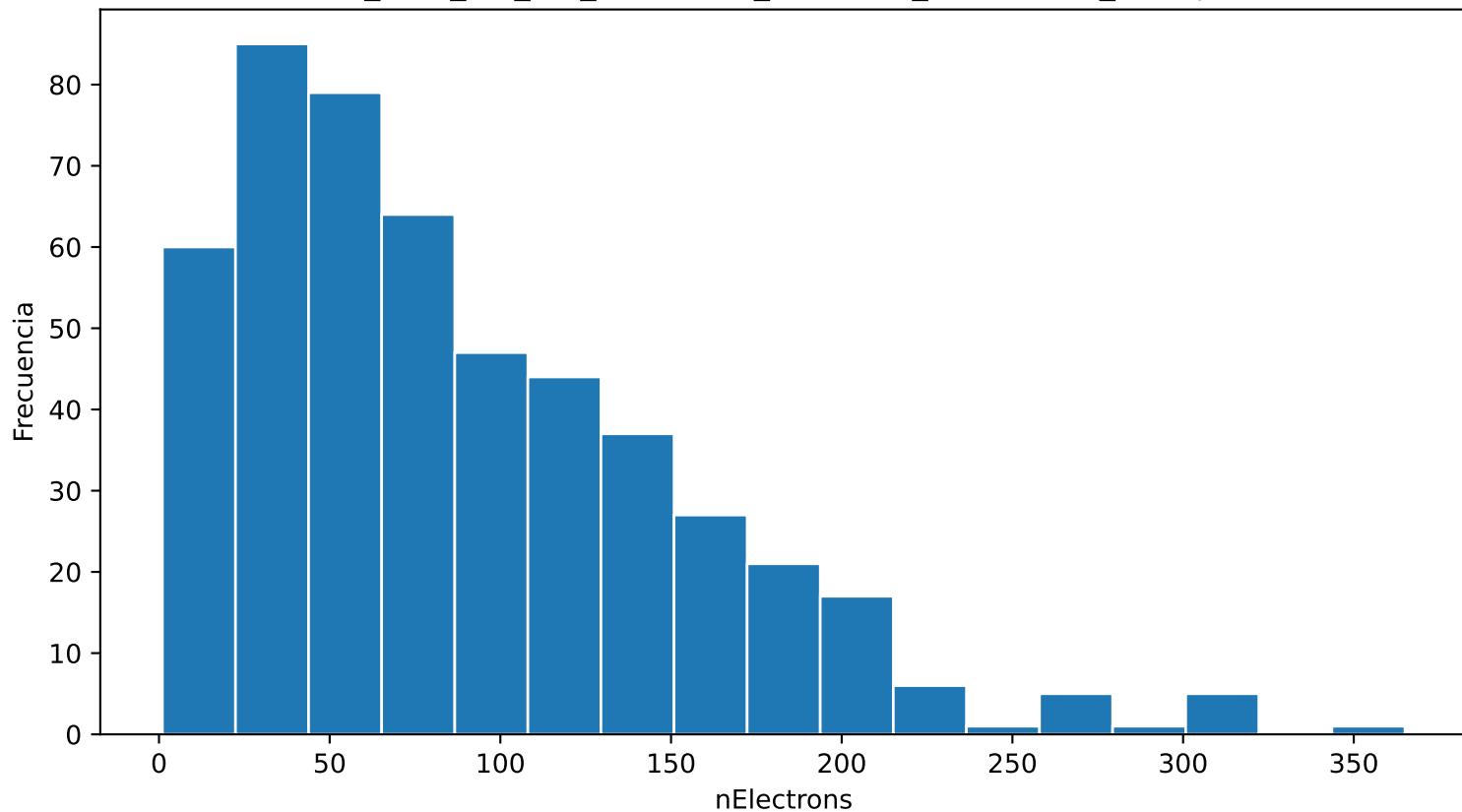
Distribución de nElectrons ar_99.0_cf4_1.0_40.0kVcm_1.000bar_0.0872mm_500npe
