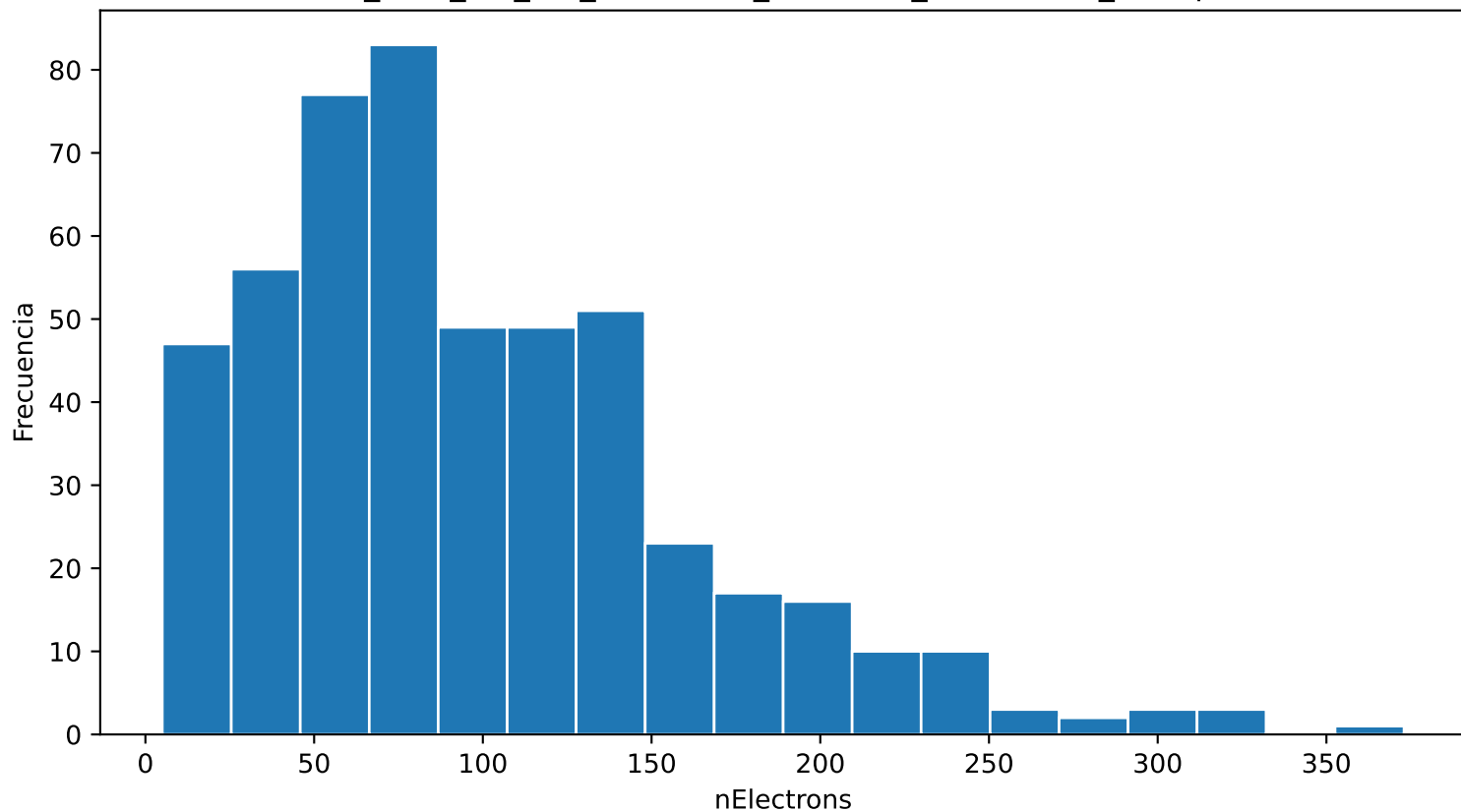
Distribución de nElectrons ar_99.0_cf4_1.0_60.0kVcm_1.000bar_0.0452mm_500npe
