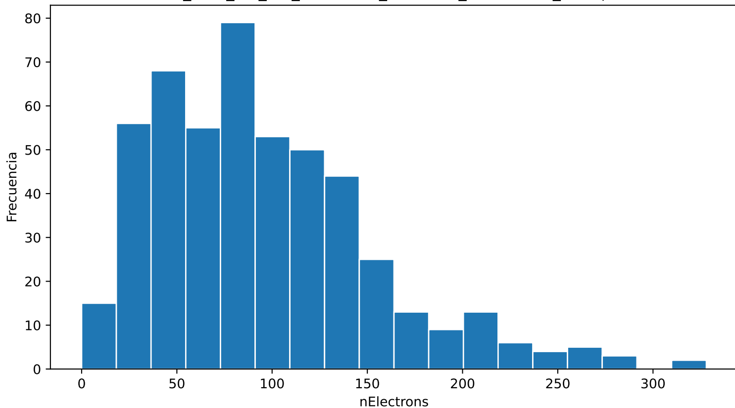
Distribución de nElectrons ar_99.0_cf4_1.0_70.0kVcm_1.000bar_0.0362mm_500npe
