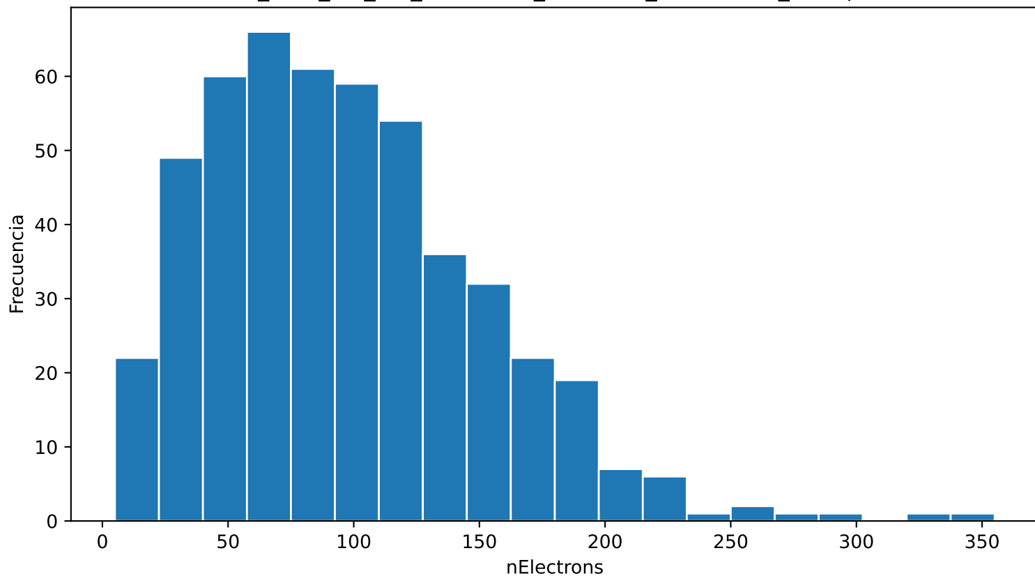
Distribución de nElectrons ar_99.0_cf4_1.0_80.0kVcm_1.000bar_0.0302mm_500npe
