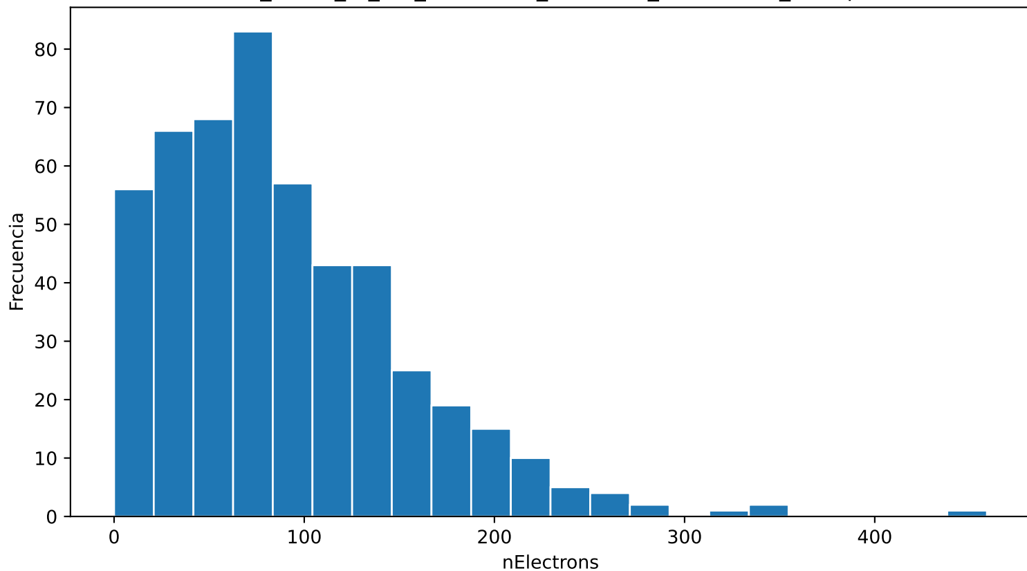
Distribución de nElectrons cf4_100.0_ar_0.0_70.0kVcm_1.000bar_0.0559mm_500npe
