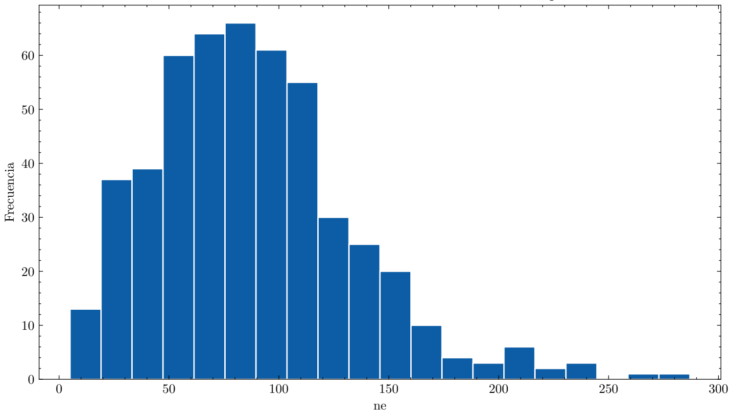
Distribución de ne ar_100.0_cf4_0.0_110.0kVcm_1.000bar_0.0199mm_500npe
