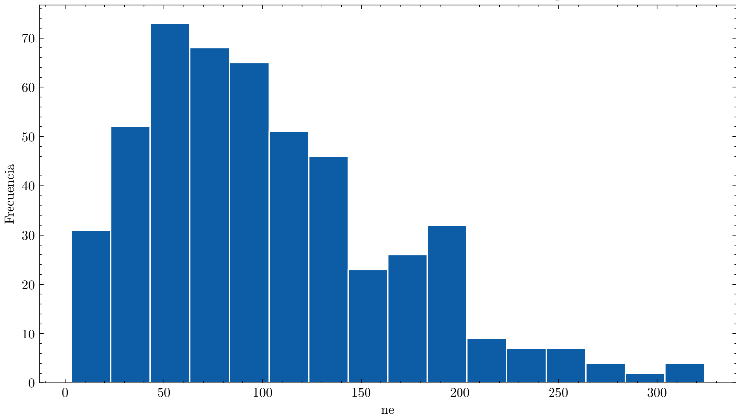
Distribución de ne ar_100.0_cf4_0.0_70.0kVcm_1.000bar_0.0364mm_500npe
