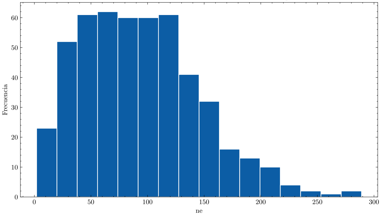
Distribución de ne ar_100.0_cf4_0.0_90.0kVcm_1.000bar_0.0258mm_500npe
