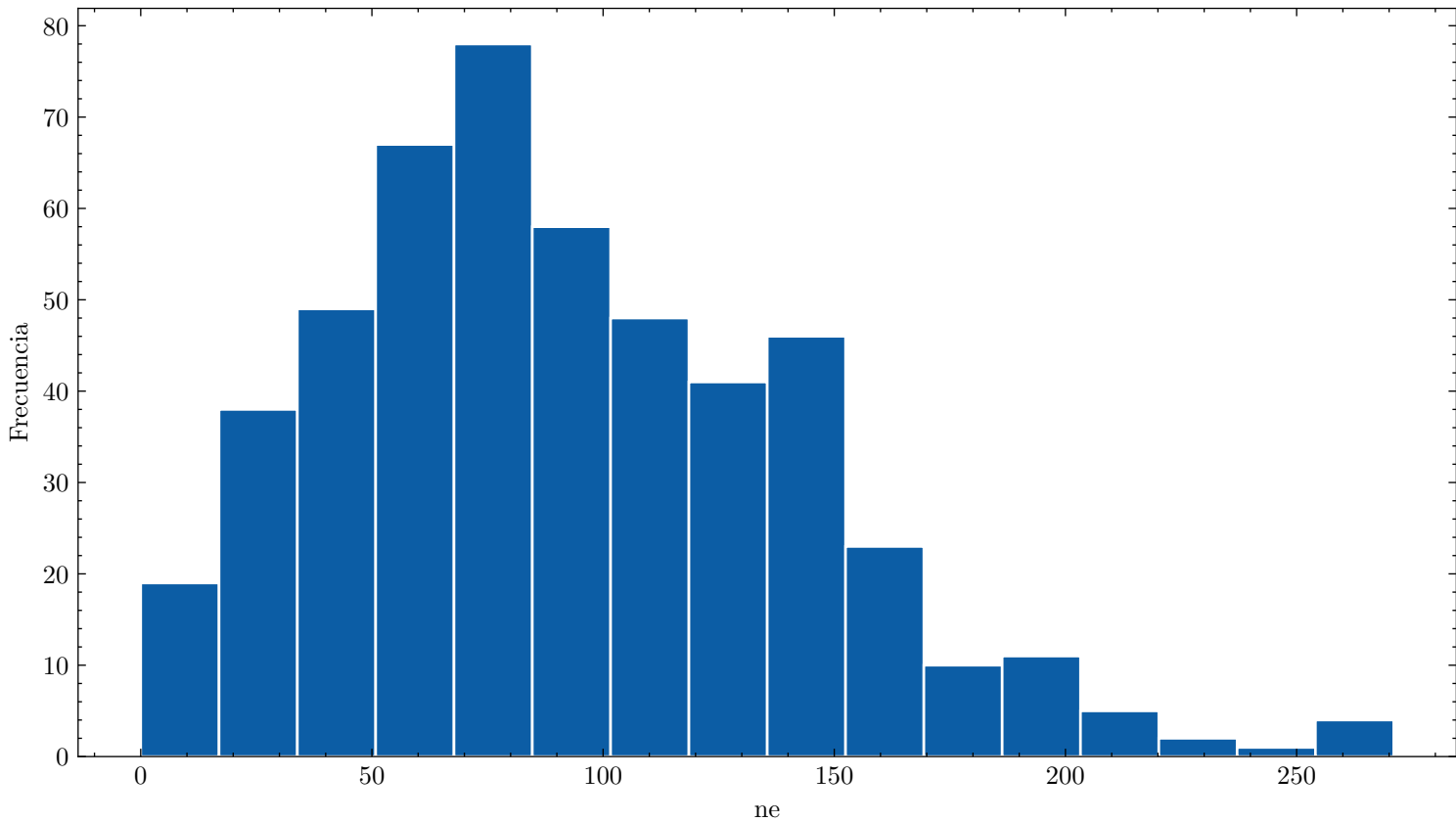
Distribución de ne ar_33.0_cf4_67.0_110.0kVcm_1.000bar_0.0230mm_500npe
