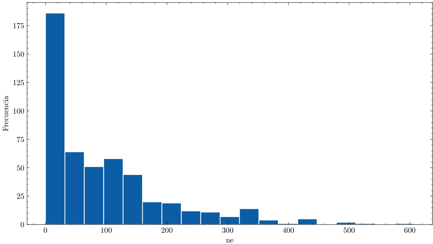
Distribución de ne ar_33.0_cf4_67.0_40.0kVcm_1.000bar_0.2255mm_500npe
