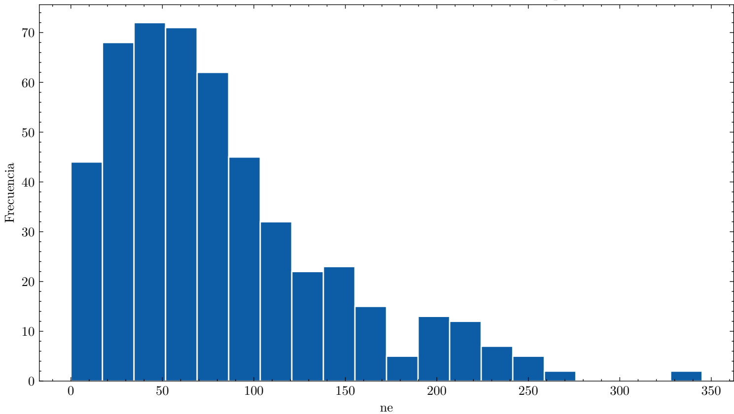
Distribución de ne ar_90.0_cf4_10.0_40.0kVcm_1.000bar_0.0938mm_500npe
