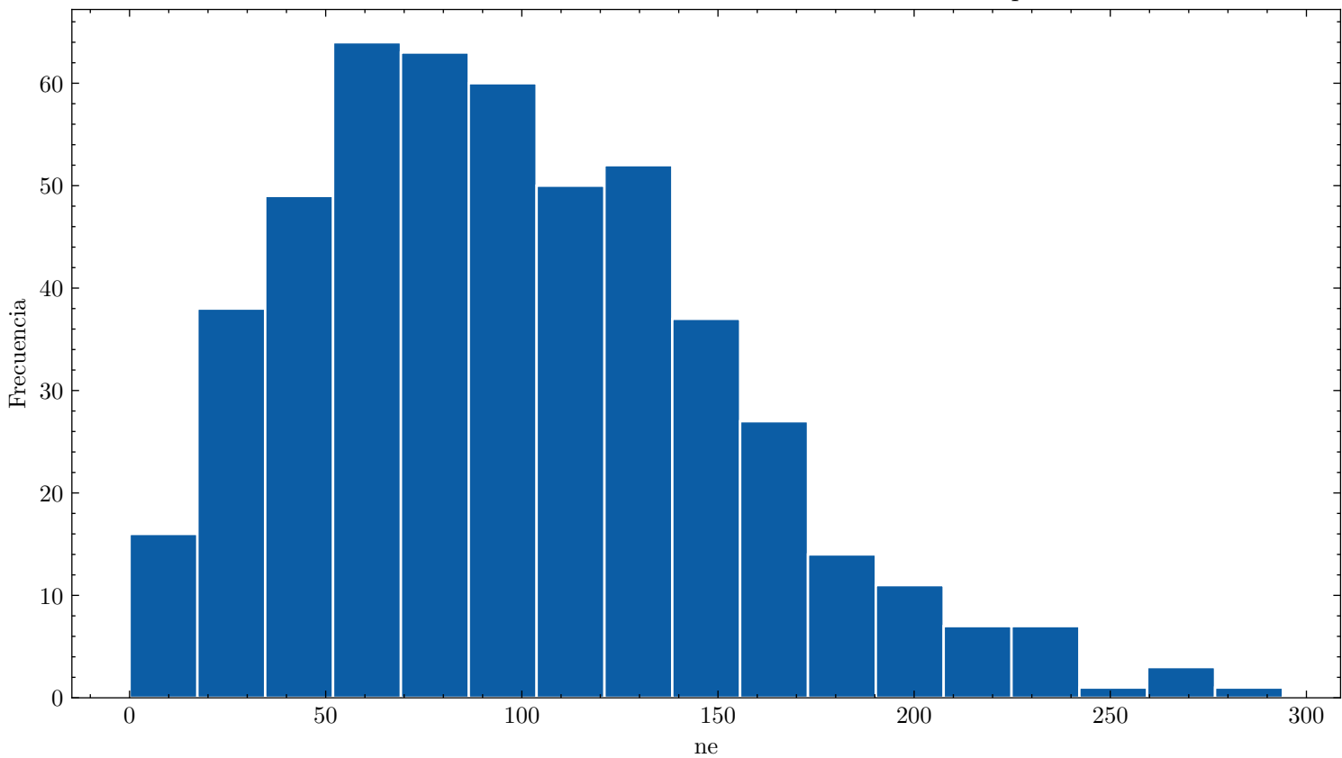
Distribución de ne ar_90.0_cf4_10.0_90.0kVcm_1.000bar_0.0267mm_500npe
