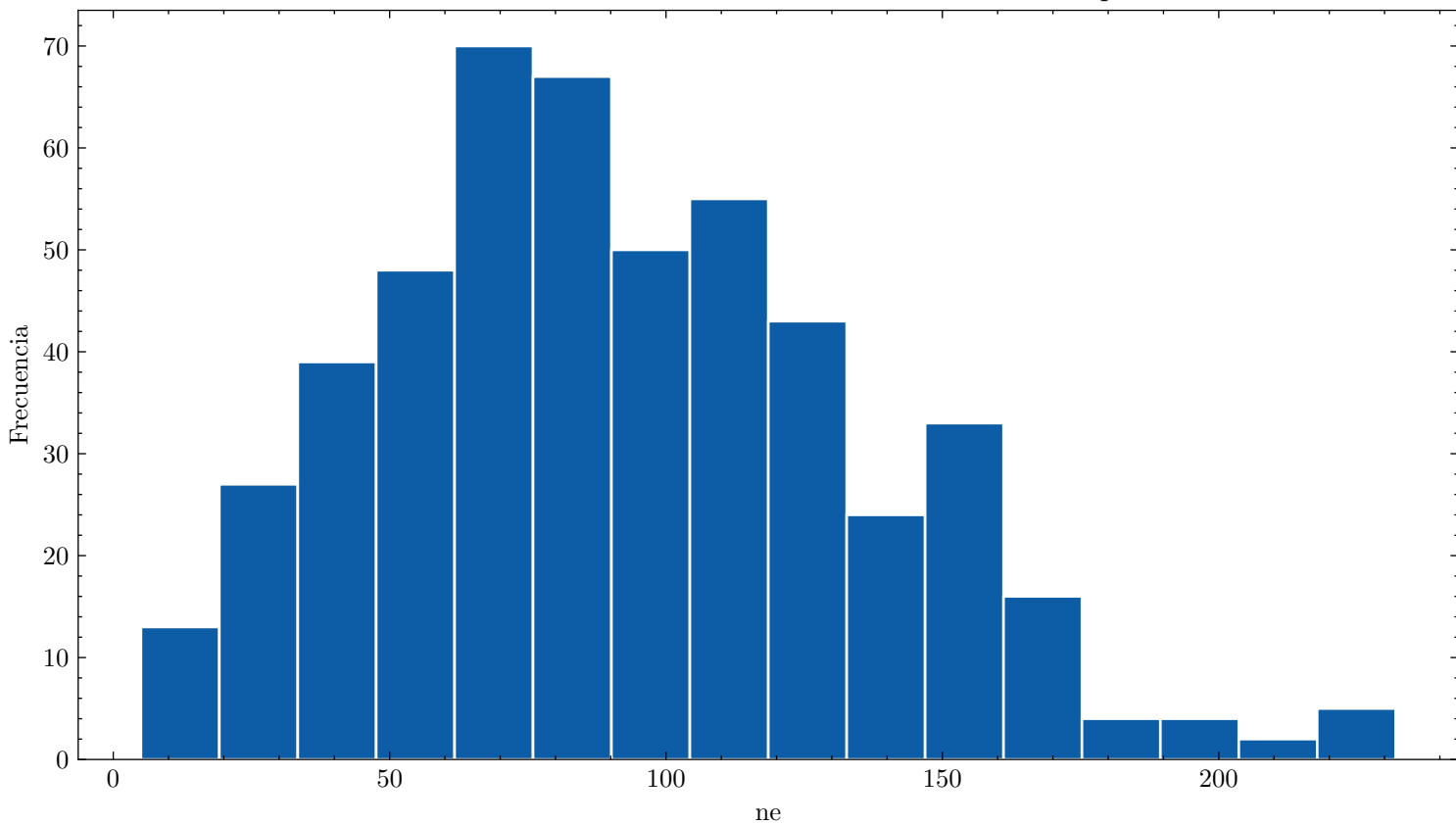
Distribución de ne ar_95.0_cf4_5.0_110.0kVcm_1.000bar_0.0202mm_500npe
