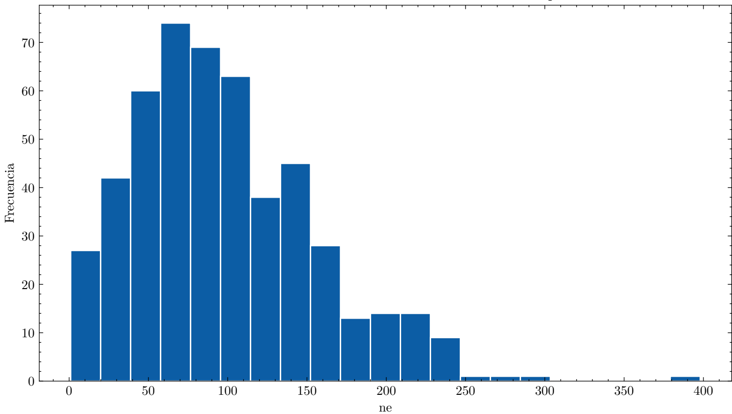
Distribución de ne ar_95.0_cf4_5.0_70.0kVcm_1.000bar_0.0369mm_500npe
