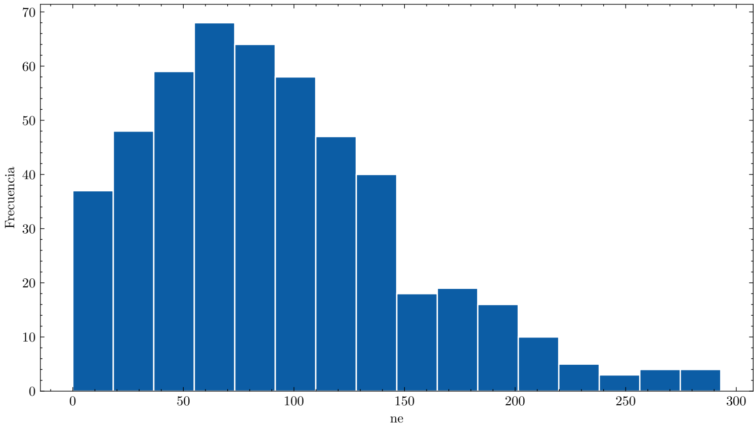
Distribución de ne cf4_100.0_ar_0.0_90.0kVcm_1.000bar_0.0347mm_500npe
