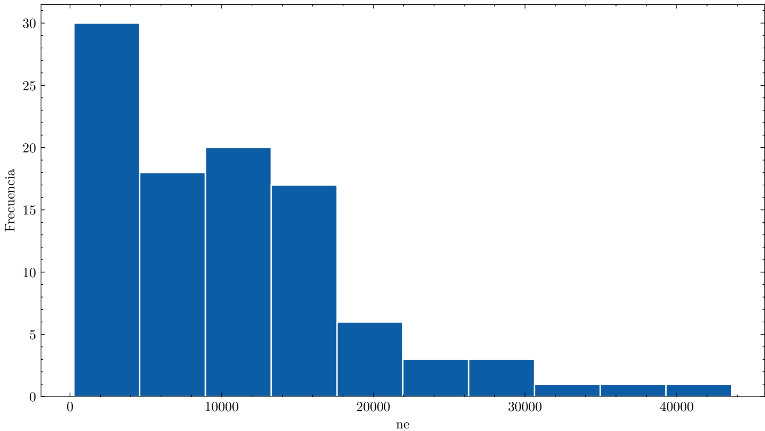
Distribución de ne ar_0.0_n2_100.0_80.0kVcm_1.000bar_0.2124mm_100npe
