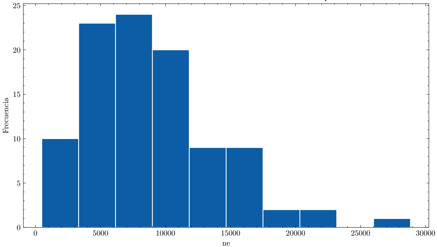
Distribución de ne ar_90.0_n2_10.0_70.0kVcm_1.000bar_0.0832mm_100npe
