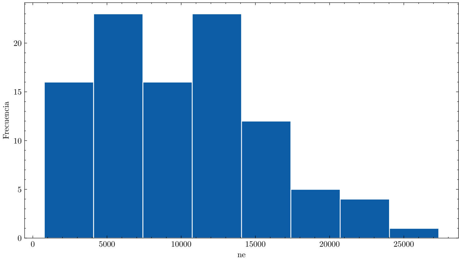
Distribución de ne ar_99.0_n2_1.0_70.0kVcm_1.000bar_0.0731mm_100npe
