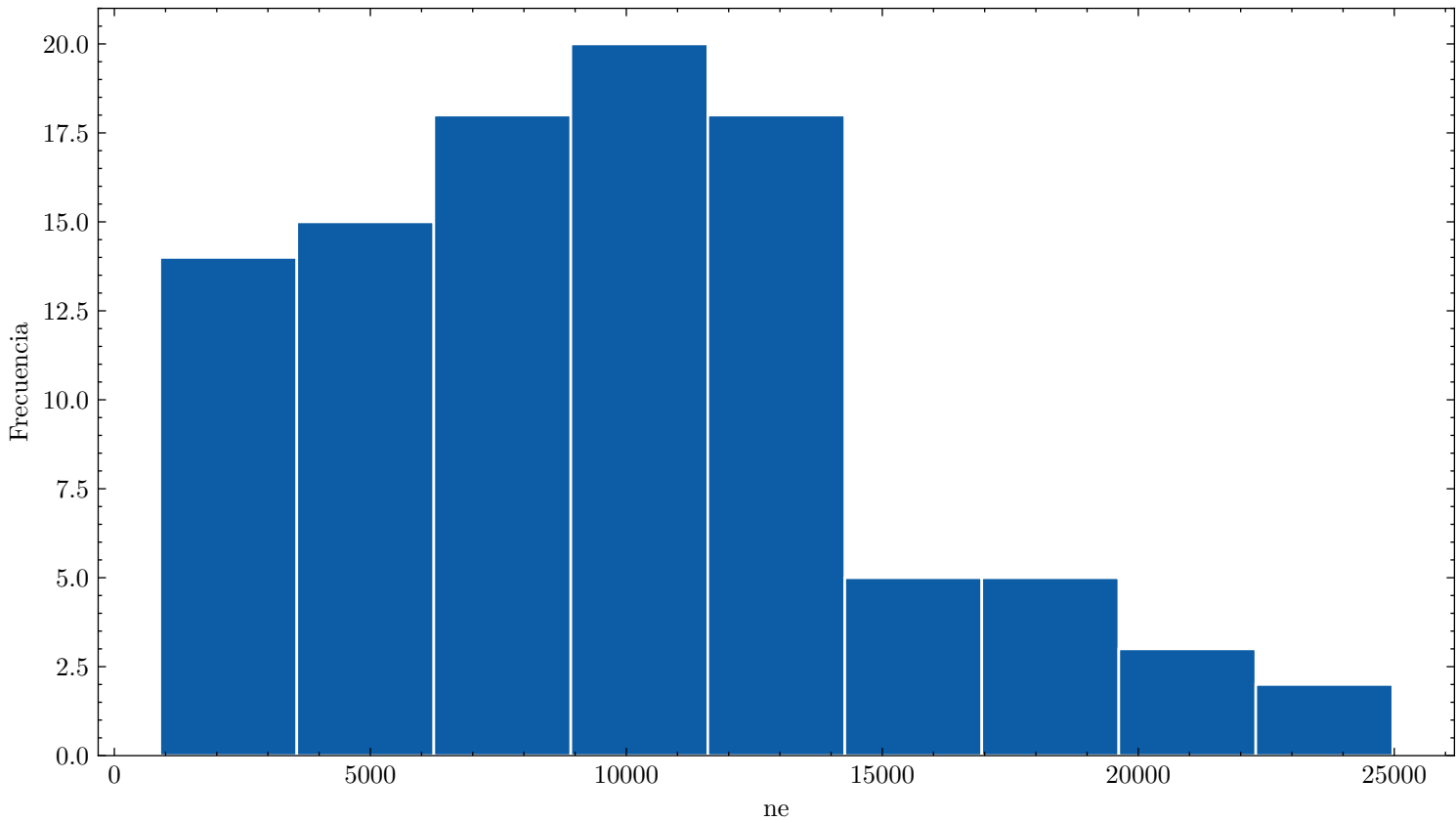
Distribución de ne ar_99.0_n2_1.0_80.0kVcm_1.000bar_0.0608mm_100npe
