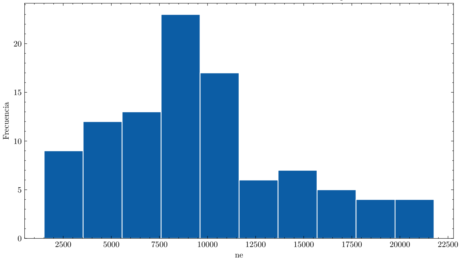
Distribución de ne ar_99.0_n2_1.0_90.0kVcm_1.000bar_0.0519mm_100npe
