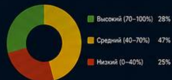
Консенсус по структурам (распределение)
