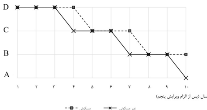
شکل ۱۹-۲-۱: زمان‌بندی الزام دستیابی به رده انرژی در ساختمان‌های جدیدالاحداث
