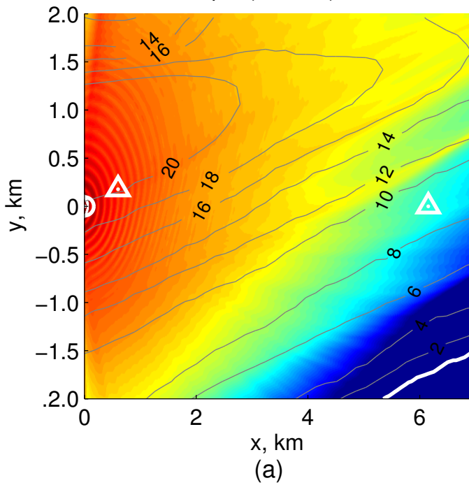
Ample ( z = 9 m), dB
