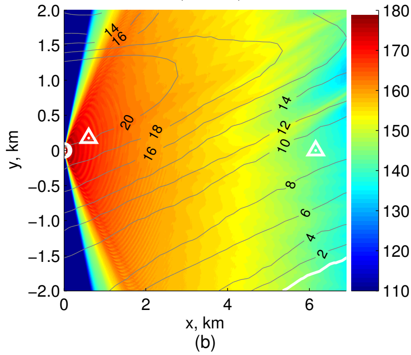
MPE ( z = 9 m), dB
