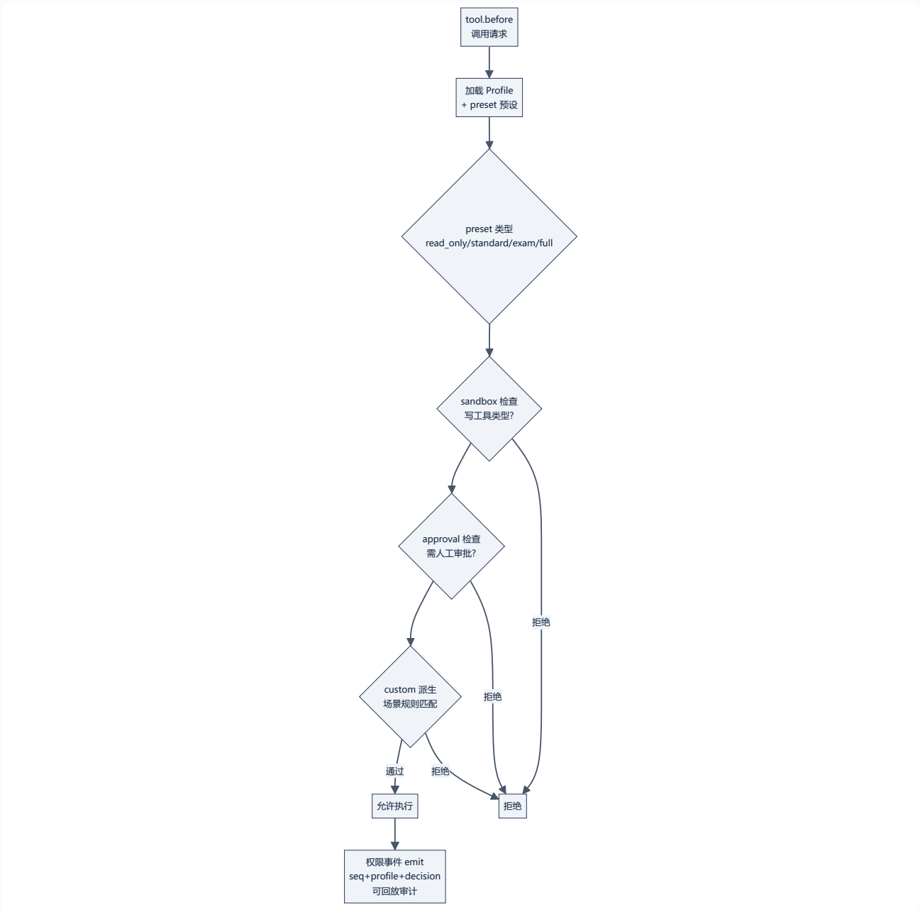
图 21 • 权限双开关 (sandbox+approval+custom)
