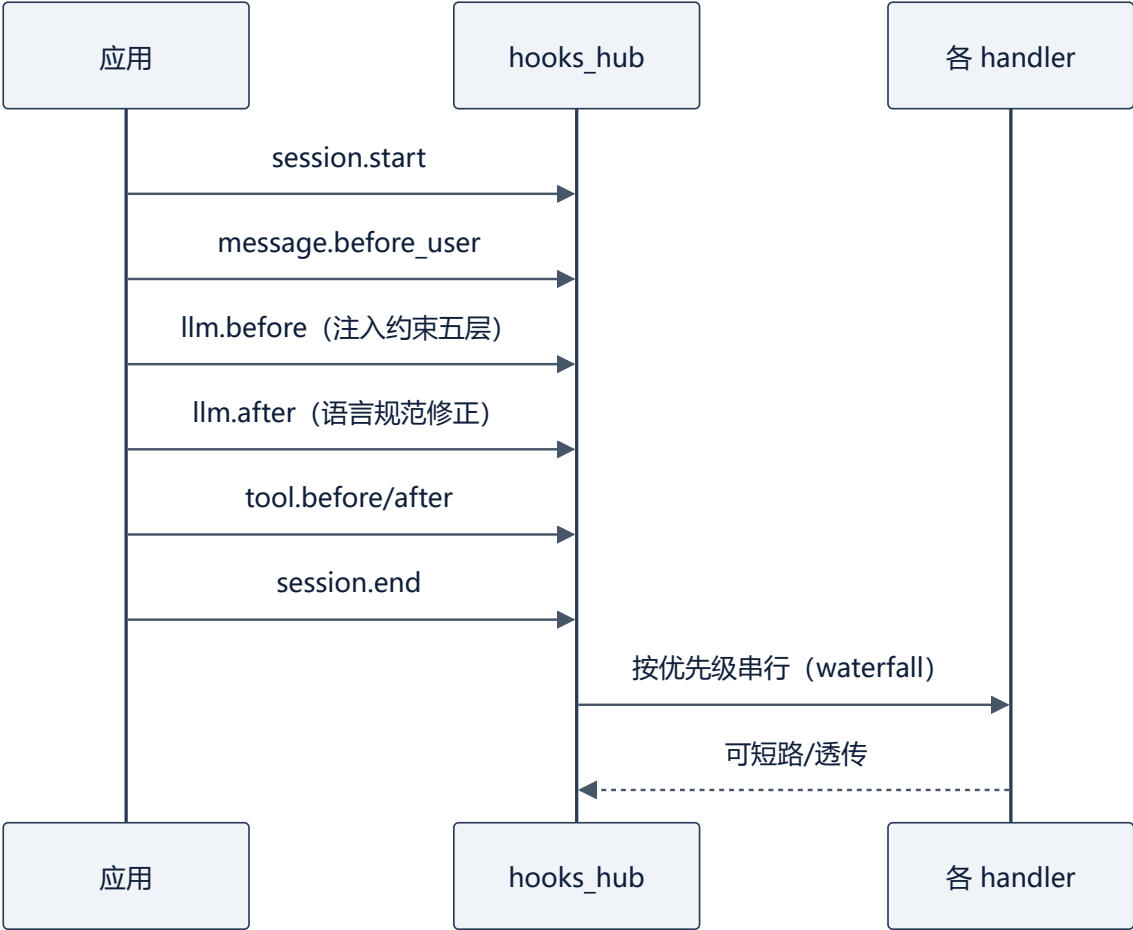
图 17 • hooks 事件链 (横切关注点)
