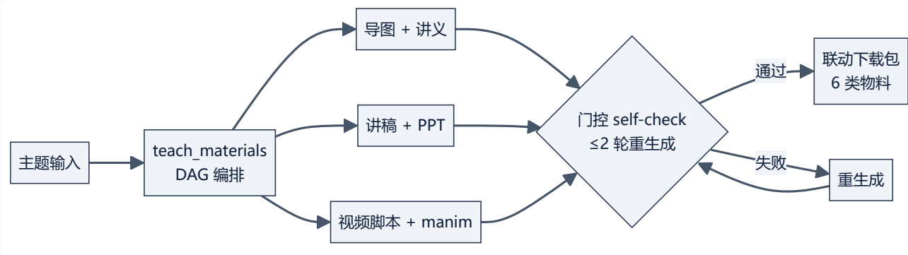
图 26 • 物料流水线 material_pipeline
