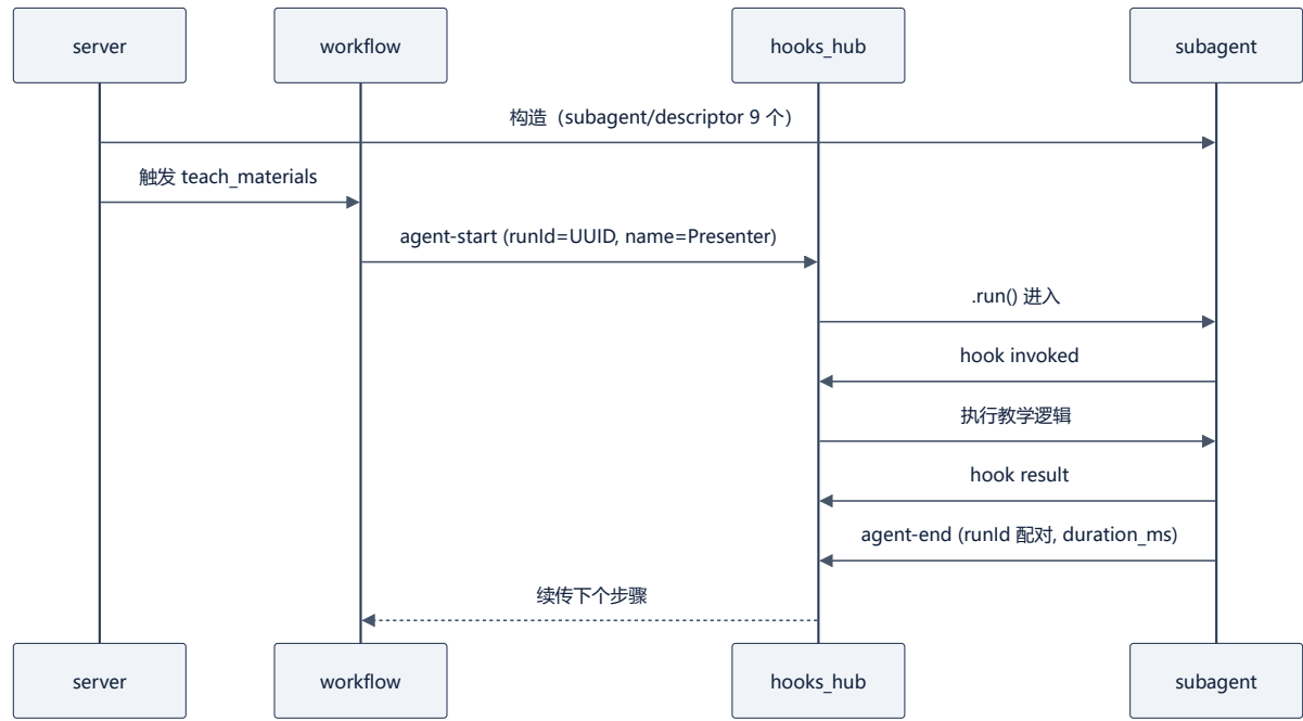
图 26 • 物料流水线 material_pipeline
