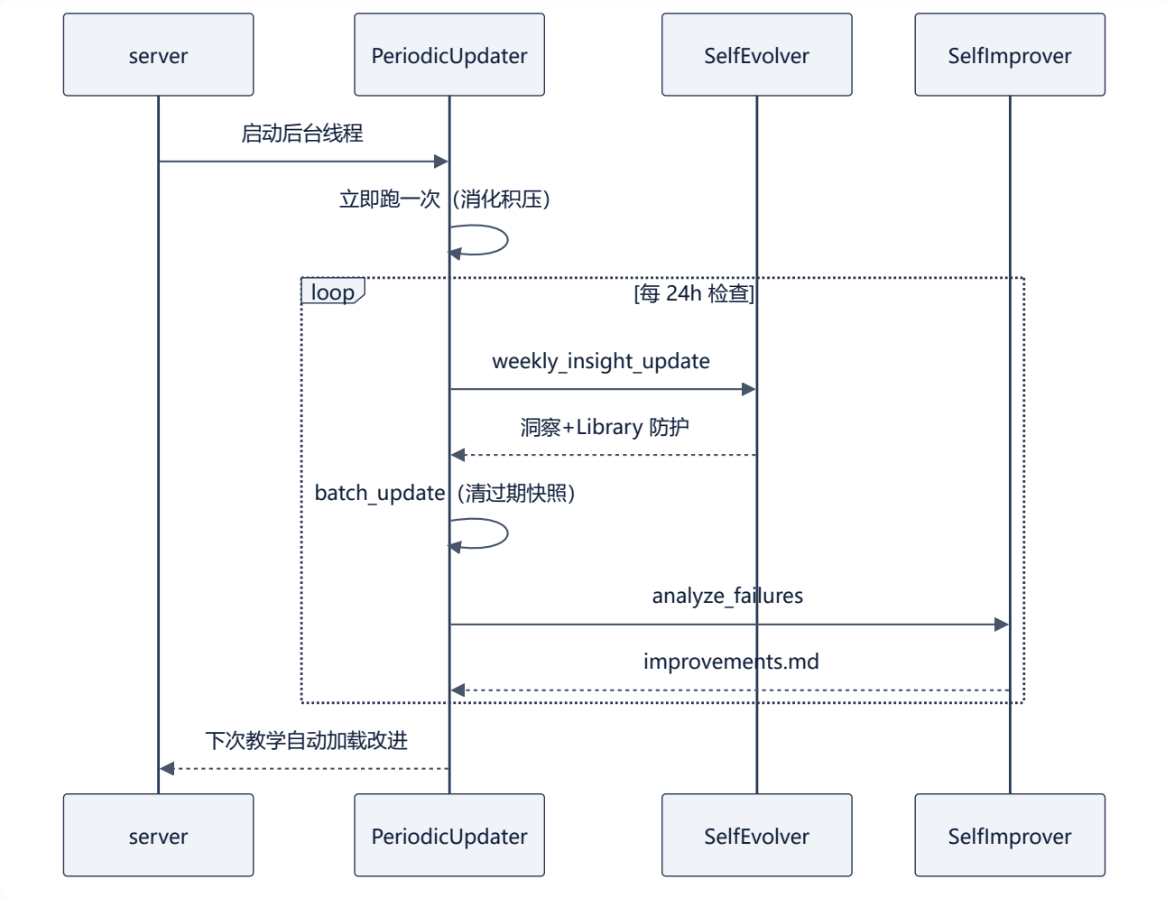
图 15 • 周期自我更新调度 (periodic)
