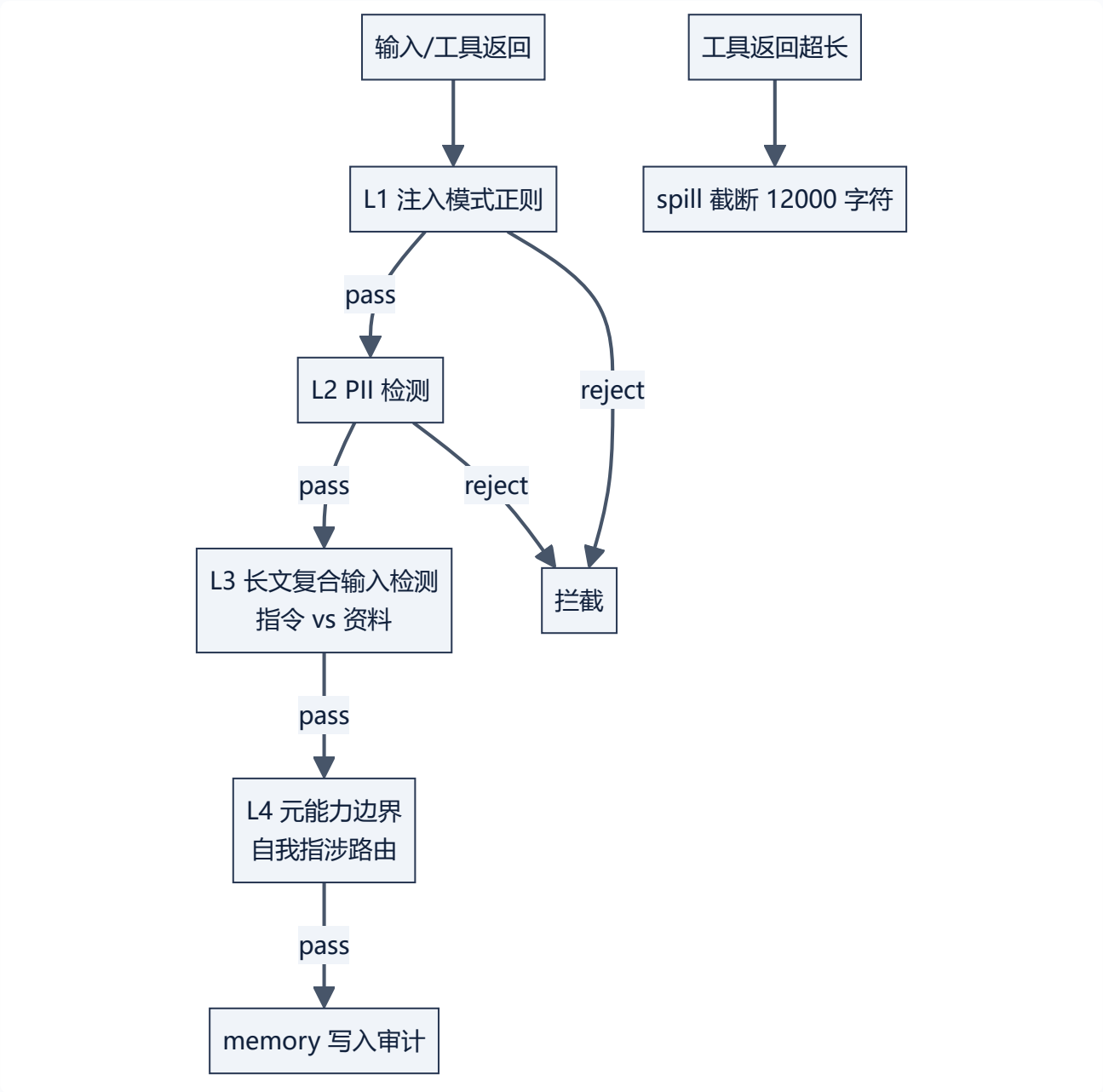
图 19 • spill 防护（上下文溢出+注入防御）
