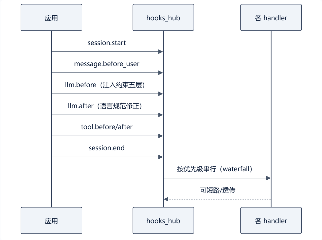
图 17 • hooks 事件链 (横切关注点)
