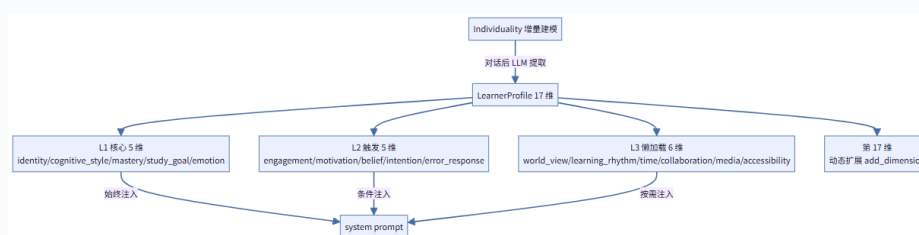
图 10 • 17 维学生画像正交模型
