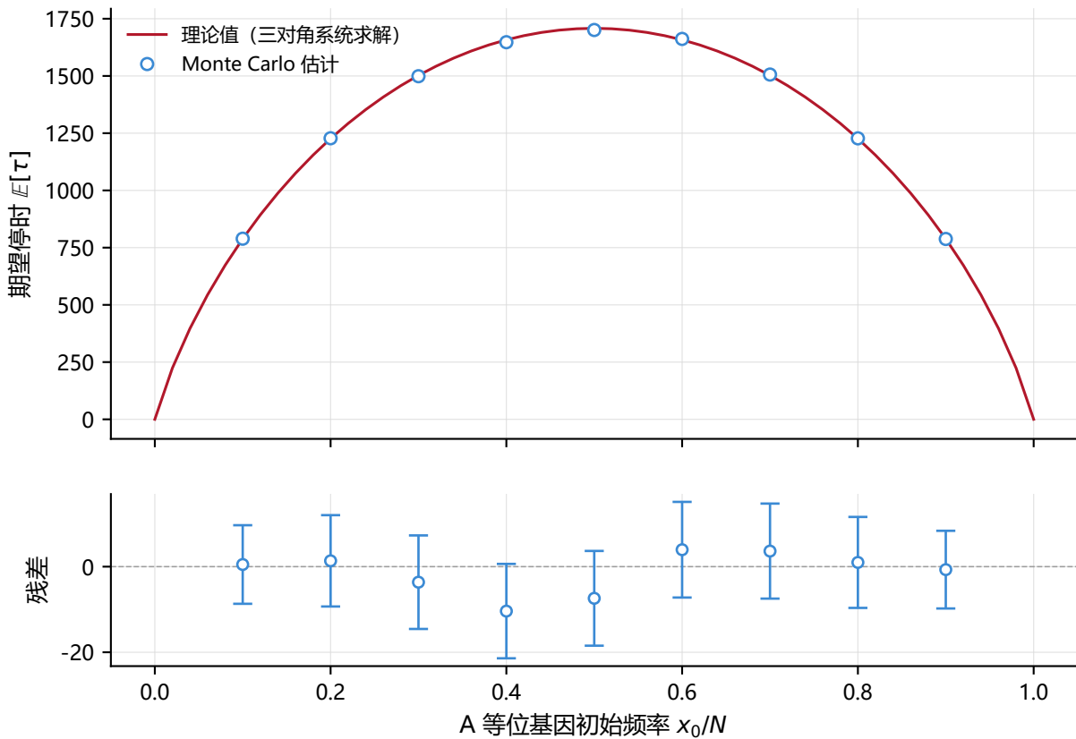
停时期望：Monte Carlo 与理论解对比 ( N = 50 )
