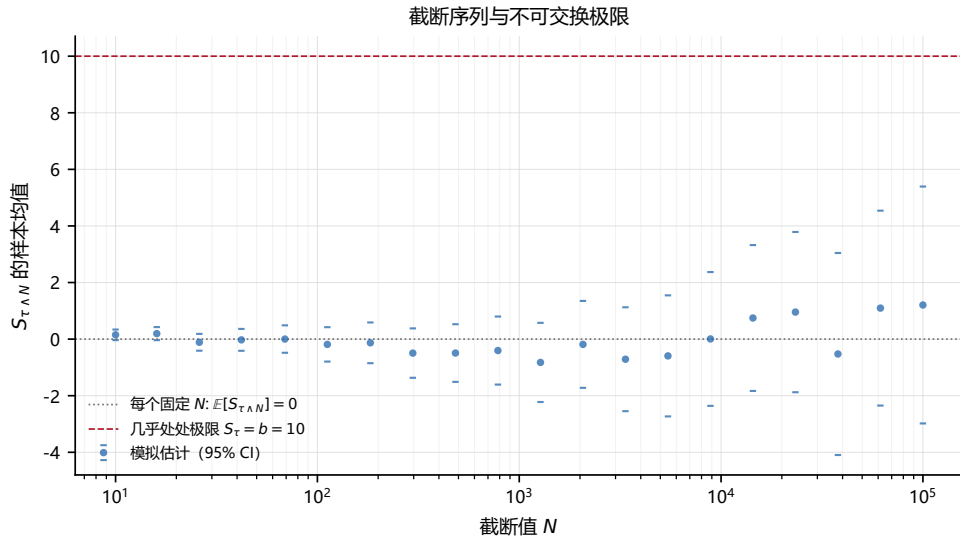
Figure 8: 截断序列与不可交换极限。对每个固定 N ，OST 给出 \mathbb{E}[S_{\tau \wedge N}] = 0 （灰色线）；但随机变量本身几乎处处收敛到 S_\tau = b = 10 （红色虚线）。样本均值在大 N 下方差显著增大，说明一致可积性缺失时不能将极限与期望交换。
