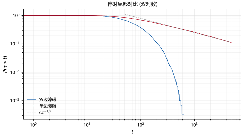
Figure 9: 停时生存函数 \mathbb{P}(\tau > t) 的双对数图。双边停时为轻尾， \mathbb{E}[\tau] < \infty ；单边停时呈 Ct^{-1/2} 型重尾， \mathbb{E}[\tau] = \infty 。重尾性是 OST 条件 3 失效的微观原因。
