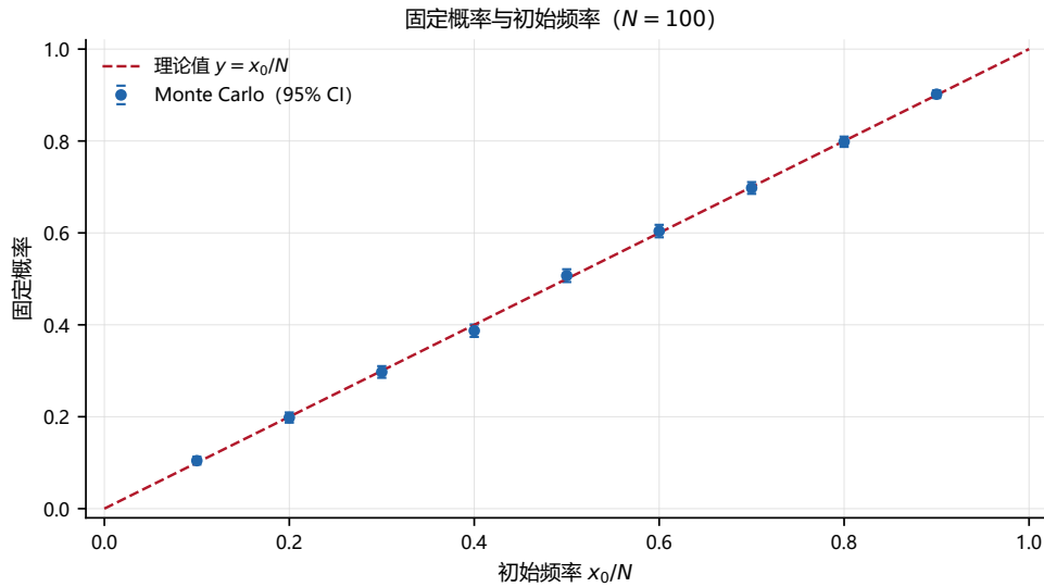
Figure 2: 固定概率与初始频率的关系 ( N = 100 )。散点为 Monte Carlo 估计 (5000 条路径 \times 9 个初始频率)，误差棒为 95% 置信区间。红色虚线为理论值 y = x_0/N ，是 OST 的直接推论。模拟与理论高度吻合，所有误差棒均跨越对角线。
