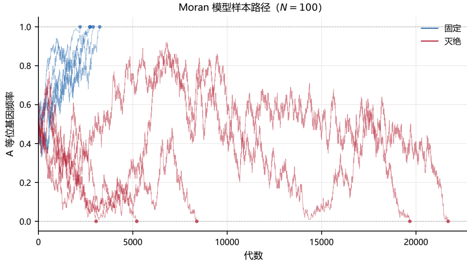
Figure 1: Moran 模型基因频率轨迹 ( N = 100 , 初始频率 0.5)。蓝色路径表示最终固定 (A 取代 a)，红色路径表示最终灭绝 (a 取代 A)。每条轨迹为锯齿状随机游走，最终被 0 或 1 吸收。圆点标记停时位置。
