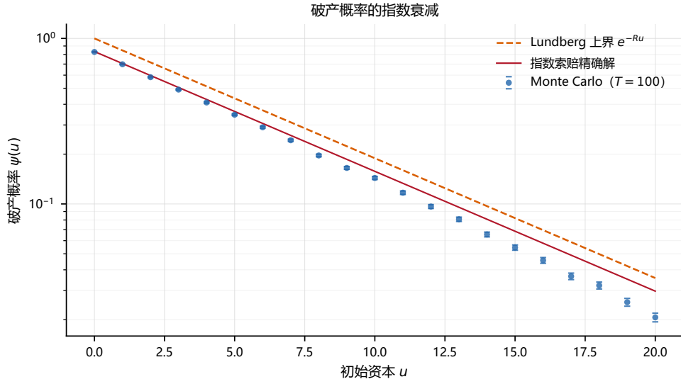
Figure 5: 破产概率的半对数图。Monte Carlo 估计（蓝色圆点， M = 50000 , T = 100 ）对应有有限视窗破产概率；红色实线为指数索赔下最终破产概率的精确解（式 (27)）。Lundberg 上界（橙色虚线）始终位于精确解之上，且在半对数图中与精确解保持近似恒定的垂直距离，反映了因子 1/(1 + \theta) 。
