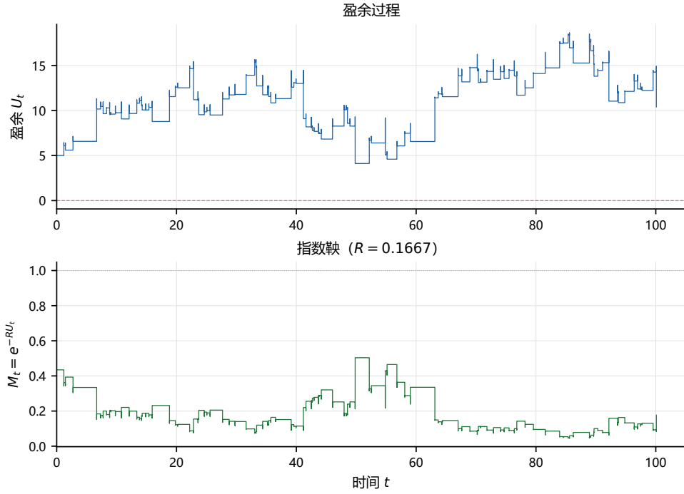
Figure 6: 同一路径的盈余过程与对应指数鞅 ( R = 0.1667 )。上子图：盈余 U_t 随时间平均上升（正向漂移 c - \lambda\mu = 0.2 ）。下子图：指数鞅 M_t = e^{-RU_t} ，无趋势，围绕初始值波动——展示了指数变换如何将一个带有漂移的过程转化为鞅。
