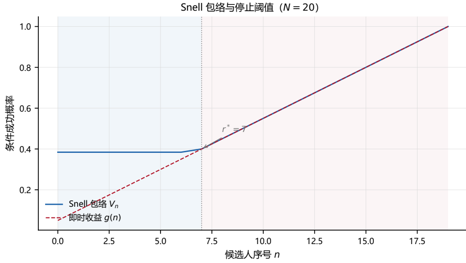
Figure 11: Snell 包络条件值 V_n 与即时 payoff g(n) 的对比 ( N = 20 )。阈值前继续等待价值高于即时收益；阈值 r^* = 7 之后两者重合，表示一旦遇到 record（历史最优）就应立即停止。 7/20 = 0.35 \approx 1/e 。
