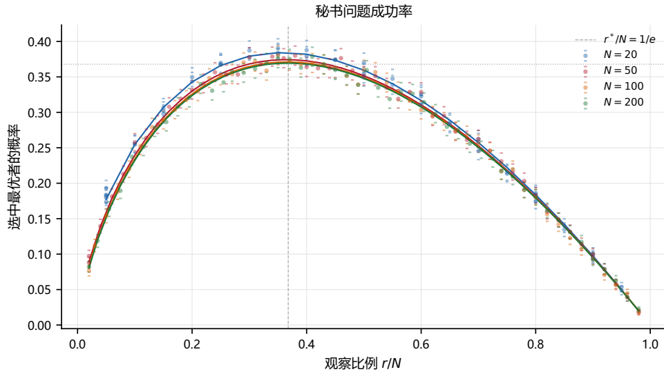
Figure 10: 秘书问题成功率与观察比例 r/N 的关系。散点为 Monte Carlo 估计（每种 N 各 5000 次试验）。实线为 N \rightarrow \infty 时的理论曲线。灰色竖虚线标记最优观察比例 r^*/N = 1/e ，灰色水平虚线标记最优成功率极限 1/e 。
