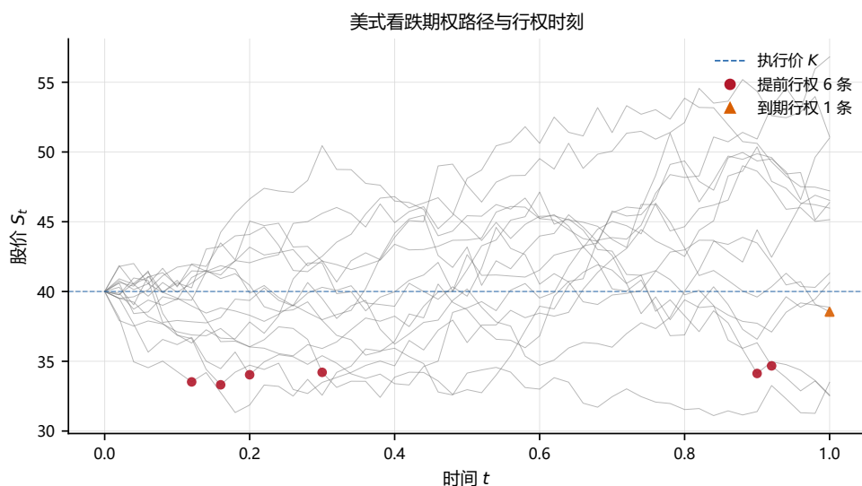
Figure 13: 几何布朗运动股价路径与 LSM 判定行权时刻（ S_0 = 40, K = 40 ）。红色圆点标记提前行权，橙色三角标记到期行权；到期价外且 payoff 为 0 的路径不额外标记。水平虚线为执行价 K 。
