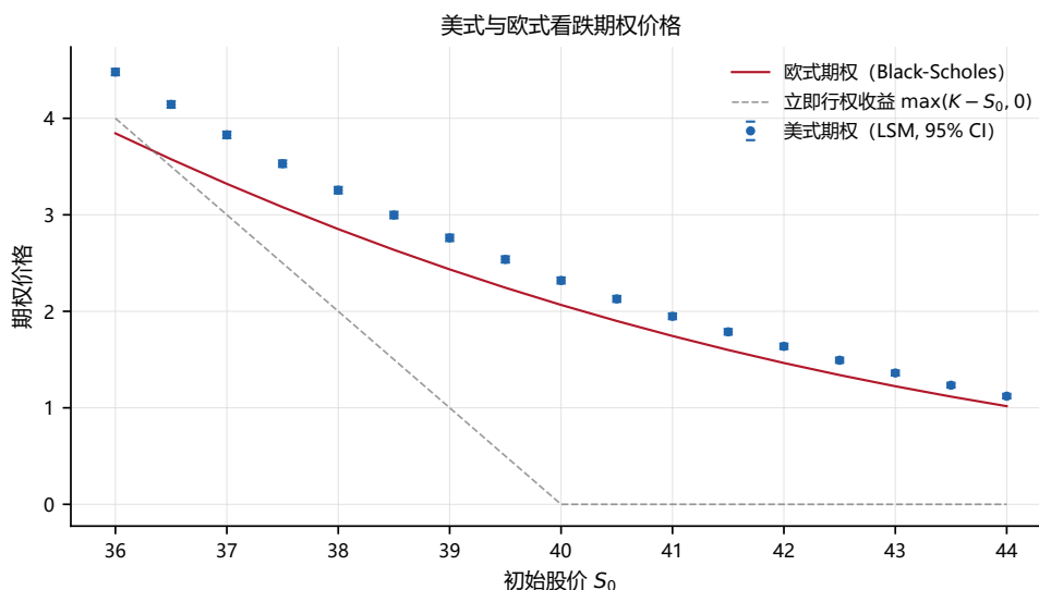
Figure 15: 美式 (LSM) 与欧式 (Black-Scholes) 看跌期权价格对比。蓝色圆点为 LSM Monte Carlo 估计 ( M = 30000 , N = 50 ), 误差棒极小 (95% CI)。红色实线为欧式 BS 公式。灰色虚线为立即行权 payoff。美式期权在所有 S_0 处均高于欧式期权, 差额即为提前行权溢价。
