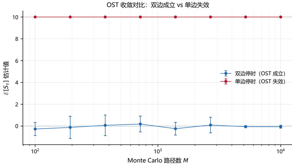
Figure 7: 双边停时与单边自然停时的 \mathbb{E}[S_\tau] Monte Carlo 估计对比。双边（蓝色）快速收敛至 OST 预测值 0（虚线）；单边（红色）命中 +b 后恒有 S_\tau = b = 10 ，因此不可能收敛到 0。
