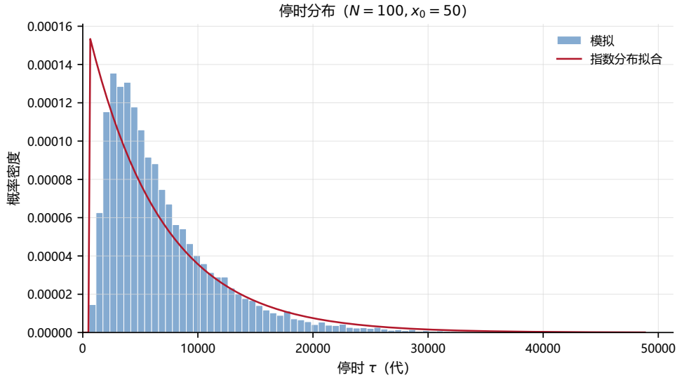
Figure 3: Moran 模型停时分布 ( N = 100, x_0 = 50 , 10000 条路径)。直方图为经验密度, 红色实线为指数分布拟合。均值为 6961 代, 中位数为 5486 代。停时分布的右偏性反映了纯漂变过程的随机性: 少数路径可能在吸收边界附近长时间“犹豫”。
