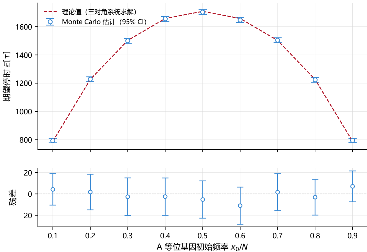
停时期望：Monte Carlo 与理论解对比 ( N = 50 )
