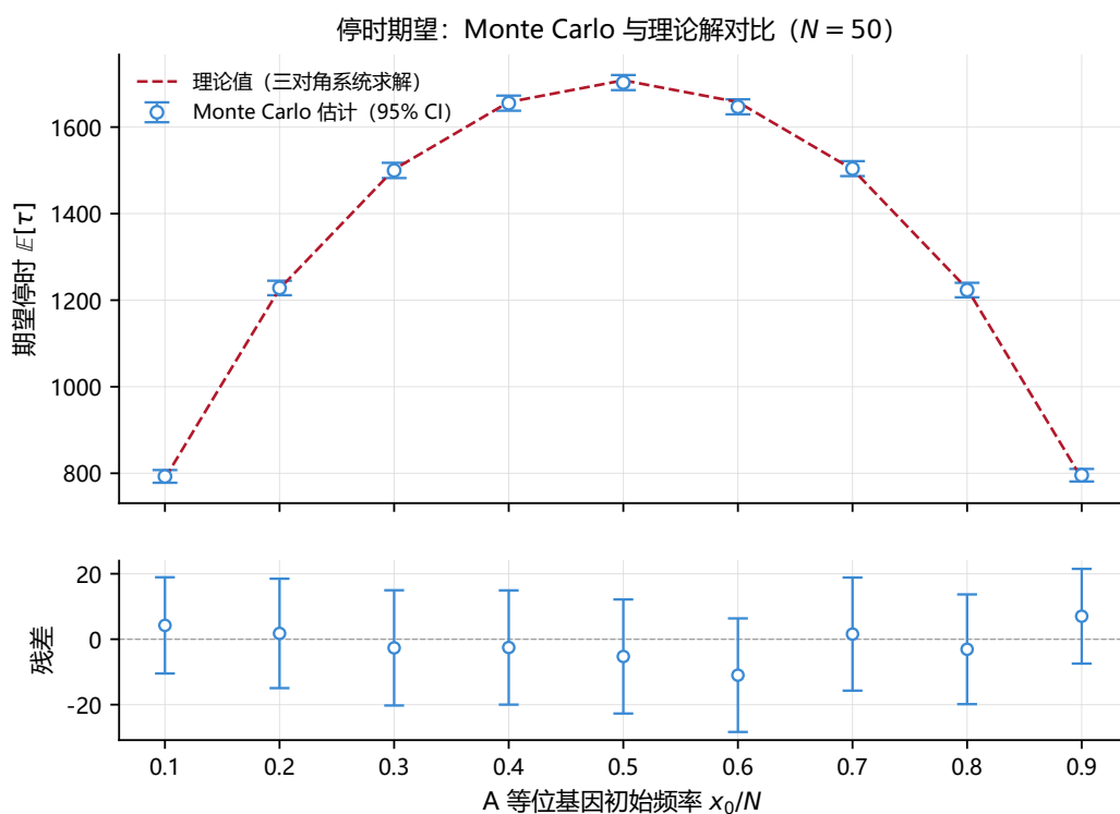
图 2.3 不同 A 等位基因初始频率下 Monte Carlo 停时均值与理论解的对比 ( N = 50 )。上图为 Monte Carlo 估计与理论值对比，蓝色圆点为 Monte Carlo 估计 (20000 条路径)，误差棒表示 95% 置信区间，红色虚线为三对角线性系统 (2.10) 给出的理论值；下图为残差 (MC - 理论)。
