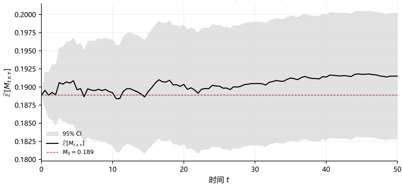
停止指数鞅的均值曲线 ( R = 0.3333 )
