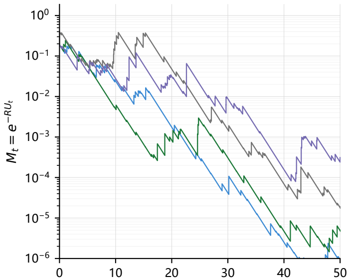
停止指数鞅的均值曲线 ( R = 0.3333 )
