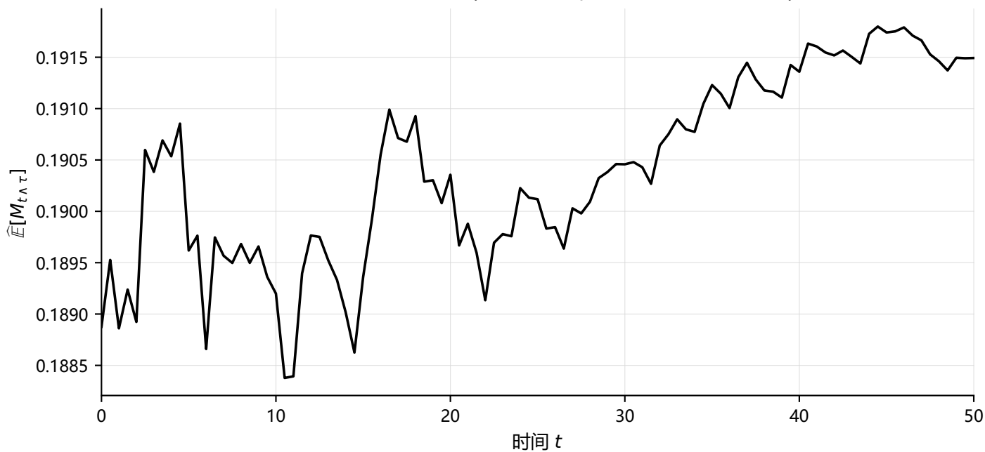
停止指数鞅的均值曲线 (理论初值 M_0 = 0.189 , R = 0.3333 )
