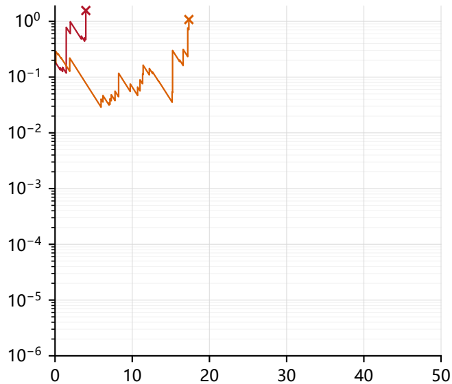
停止指数鞅的均值曲线 (理论初值 M_0 = 0.189 , R = 0.3333 )
