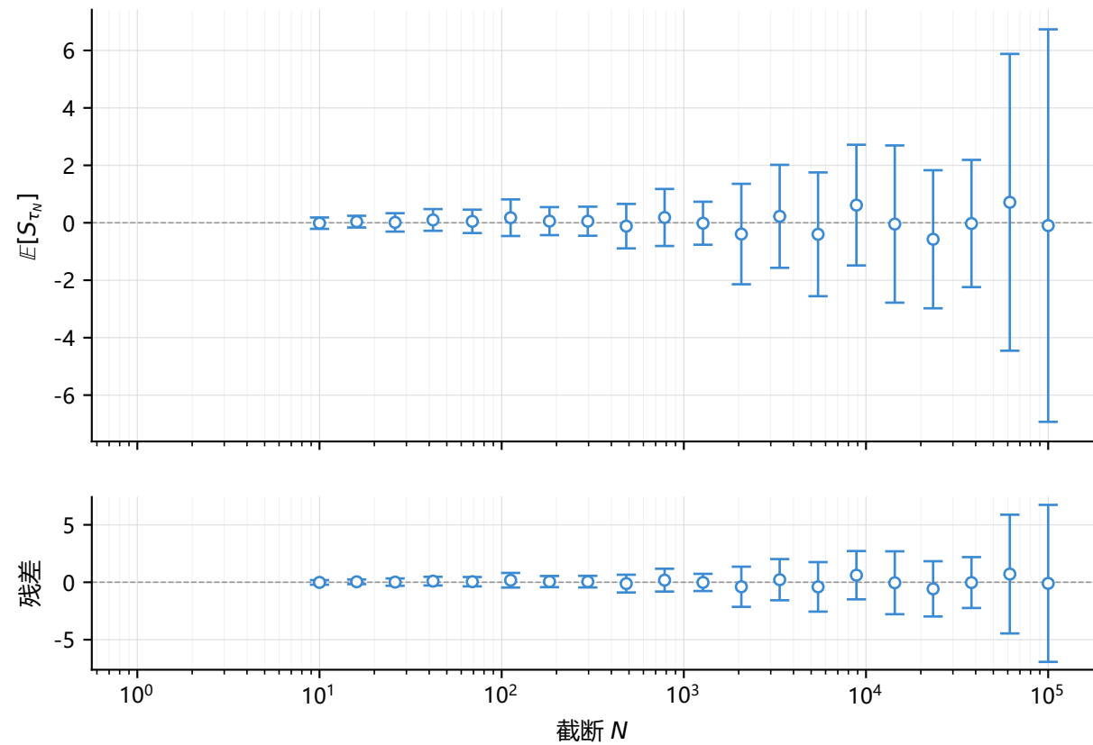
截断停时期望收敛 (单边障碍 b = 10 )
