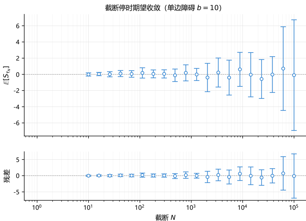
图 4.4 截断停时期望 \mathbb{E}[S_{\tau_N}] 随截断 N 的变化。上图：期望值在不同 N 下的 Monte Carlo 估计 (1000 条路径, 12 批次, 误差棒为 95% 置信区间), 灰色虚线为零线; 下图：残差面板。对所有 N , 估计值均围绕零波动, 不收敛至 b = 10 , 体现了一致可积性的缺失。
