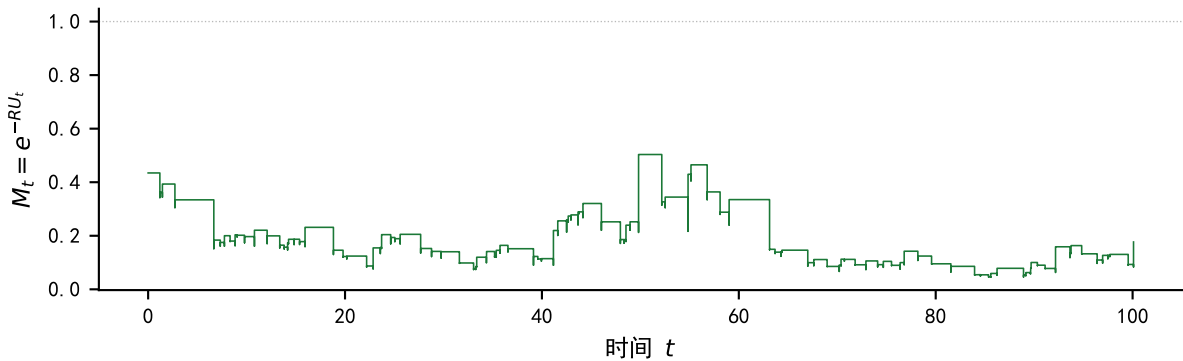
指数鞅 (调整系数 R=0.1667 )
