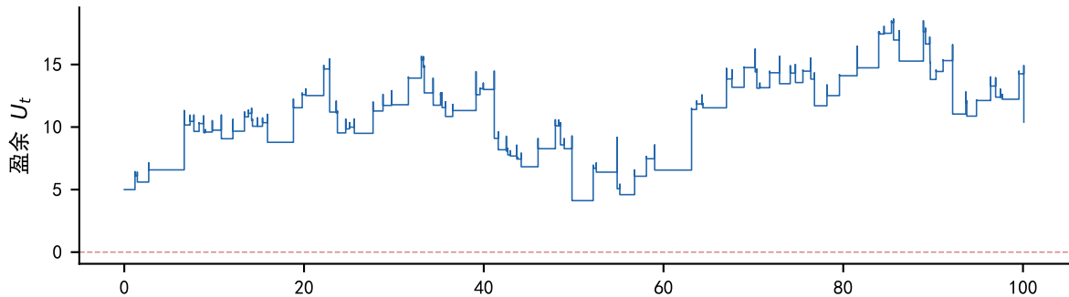
指数鞅 (调整系数 R=0.1667 )
