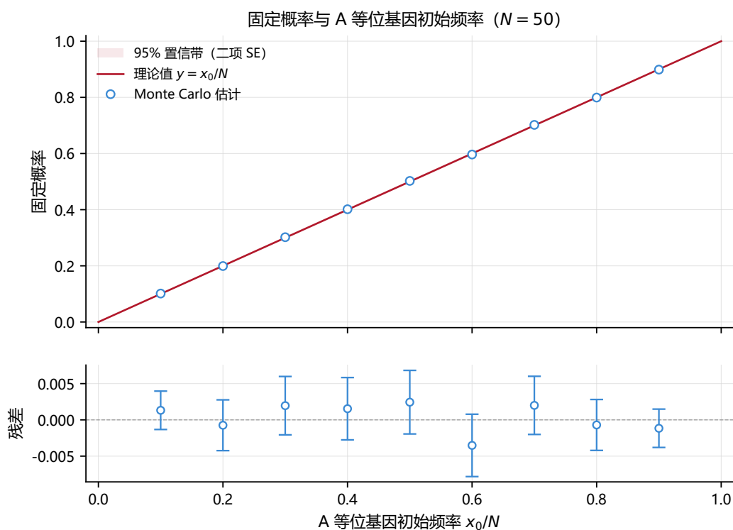
图 2.2 固定概率与 A 等位基因初始频率的关系 ( N = 50 )。上图：红色实线为理论值 y = x_0/N ，红色阴影为二项标准误给出的 95% 置信带，蓝色圆点为 Monte Carlo 估计 (50000 条路径)。下图：估计值偏离理论值的残差，误差棒为 95% 置信区间。
