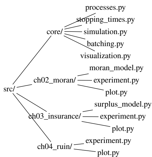
图 1.1 项目代码文件架构。核心层（ src/core/ ）提供可复用的鞅过程、停时和模拟引擎；第二、三章的实验层包含模型定义、实验脚本和绘图脚本，第四章则直接复用核心层中的对称随机游走实现。
