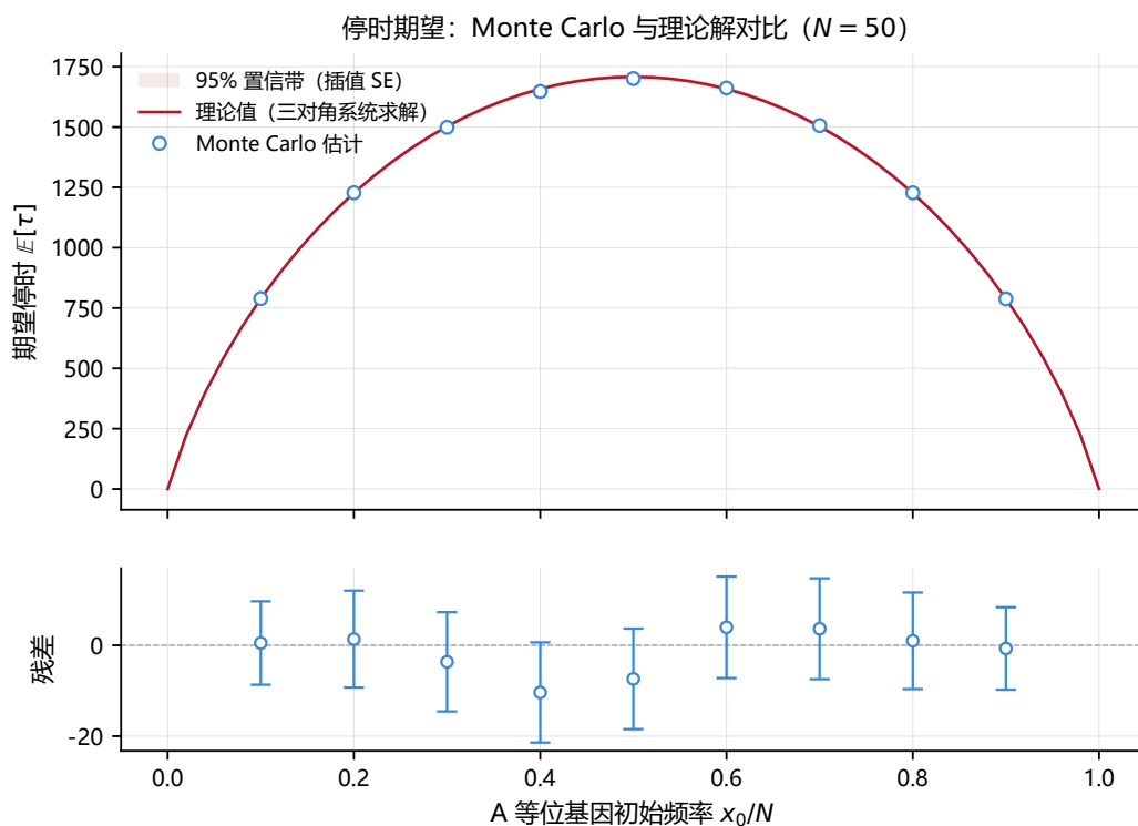
图 2.3 不同 A 等位基因初始频率下 Monte Carlo 停时均值与理论解的对比 ( N = 50 )。上图：红色实线为三对角线性系统 (2.10) 给出的理论值，红色阴影为插值 SE 给出的 95% 置信带，蓝色圆点为 Monte Carlo 估计 (50000 条路径)。下图：估计值偏离理论值的残差，误差棒为 95% 置信区间。
