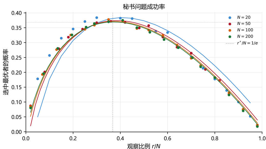
图 5.1 秘书问题成功率与观察比例 r/N 的关系。圆点为 Monte Carlo 成功率估计（每点 5000 次试验）；实线为对应的理论曲线。灰色竖虚线标记最优观察比例 r^*/N = 1/e ，灰色水平虚线标记最优成功率极限 1/e 。
