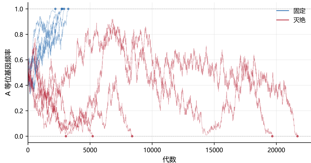
Moran 模型样本路径 ( N = 100 )
