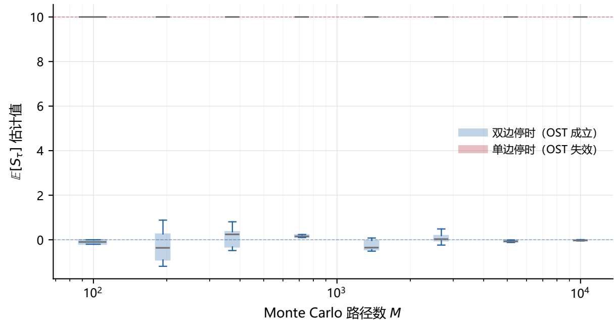
OST 收敛对比: 双边成立 vs 单边失效
