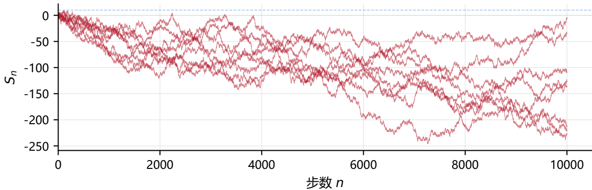
未达到 +10 的路径 (截断 N = 10000 )
