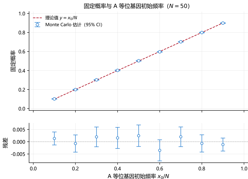
图 2.2 固定概率与 A 等位基因初始频率的关系 ( N = 50 )。上图: Monte Carlo 估计 (蓝色圆点, 50000 条路径, 误差棒为 95% 置信区间) 与理论值 y = x_0/N (红色虚线) 对比。下图: 估计值偏离理论值的残差。
