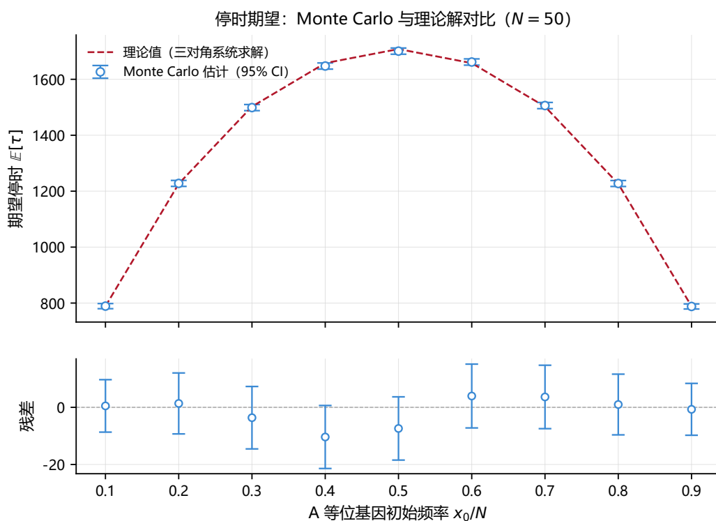
图 2.3 不同 A 等位基因初始频率下 Monte Carlo 停时均值与理论解的对比 ( N = 50 )。上图：Monte Carlo 估计（蓝色圆点，50000 条路径，误差棒为 95% 置信区间）与三对角线性系统 (2.10) 给出的理论值（红色虚线）对比。下图：估计值偏离理论值的残差。
