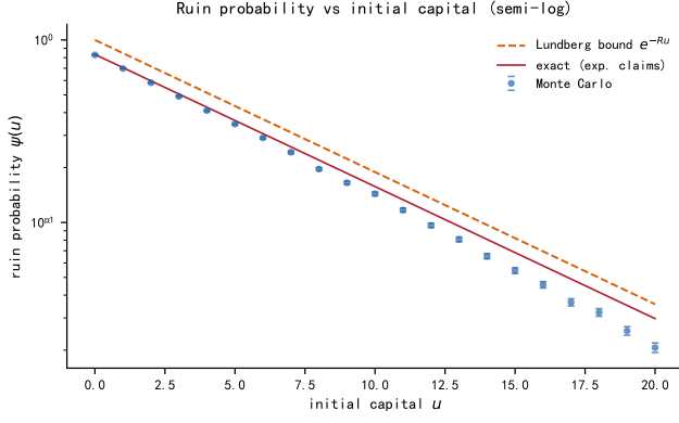
图 5. 破产概率的半对数图。Monte Carlo 估计（蓝色圆点， M = 50000 ）与指数索赔精确解（红色实线，式 (27)）在 u \leq 10 区域高度吻合。Lundberg 上界（橙色虚线）始终位于两者之上，且在半对数图中与精确解保持近似恒定的垂直距离，反映了因子 1/(1 + \theta) 。
