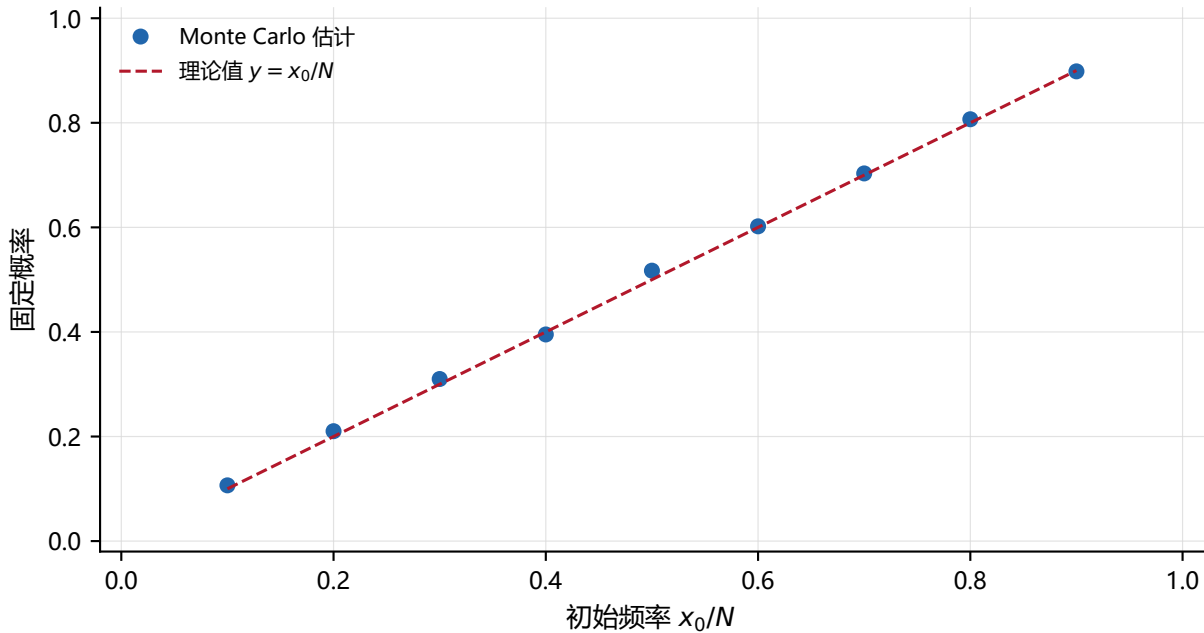
固定概率与初始频率 ( N = 50 )
