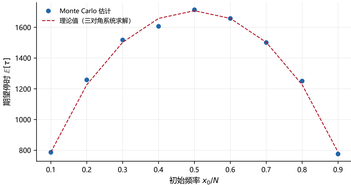
停时期望：Monte Carlo 与理论解对比 ( N = 50 )
