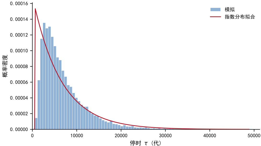
Moran 模型停时分布 ( N=100 , x_0=50 )
